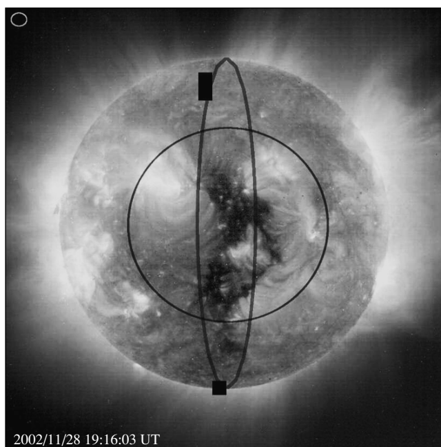
Рис. 1. Корональная дыра, наблюдавшаяся в канале \lambda 284 \text{ \AA} 28 ноября 2002 г. Место измерения фона показано на рисунке кружком в левом верхнем углу (см. п. 2.2). Указаны границы сферического сектора и круга радиусом 0.6 R_0 .
