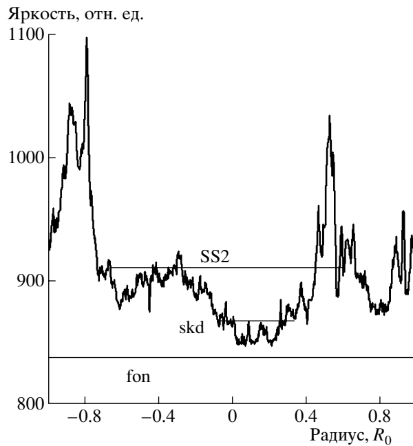
Рис. 2. Одномерное центральное сечение яркости диска 28 ноября 2002 г. Указаны некоторые используемые индексы.
