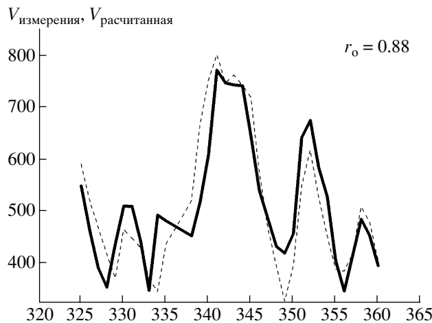
Рис. 4. Измеренные (штриховая кривая) и вычисленные (сплошная кривая) значения скорости в период с 21 ноября по 26 декабря 2003 г.
